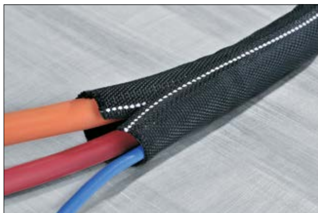
Helagaine Twist-In-FRX anvendes hvor brandsikkerhed er vigtig.
